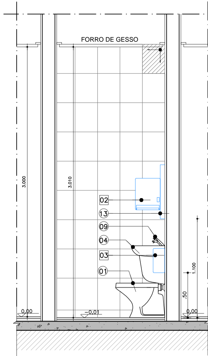
CORTE AA ESCALA 1:25 AM-01- WC PLANTÃO - TÉRREO
