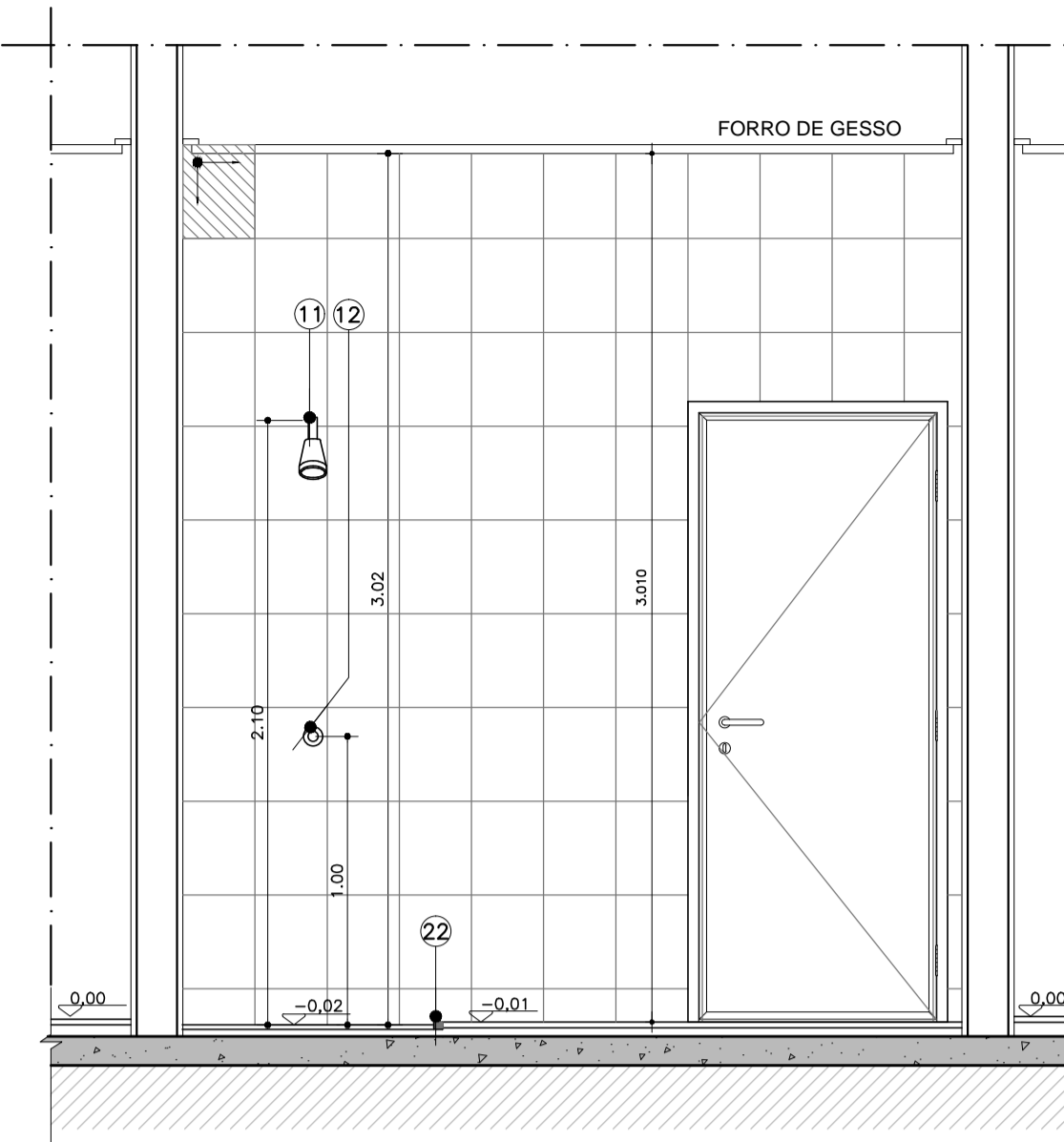
CORTE DD ESCALA 1:25 AM-01- WC PLANTÃO - TÉRREO
