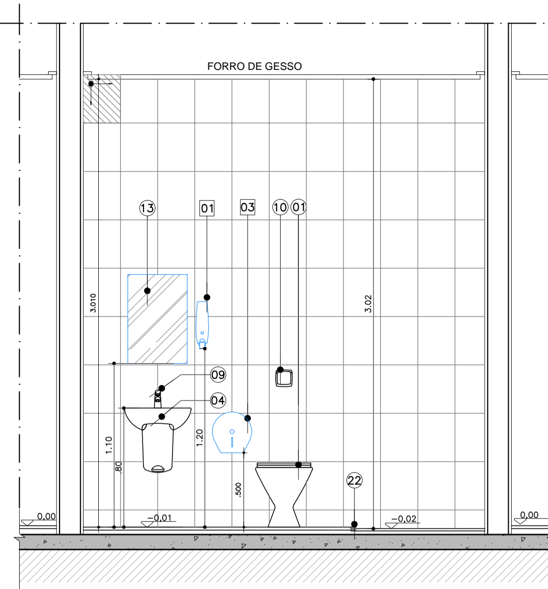
CORTE BB ESCALA 1:25 AM-01- WC PLANTÃO - TÉRREO
