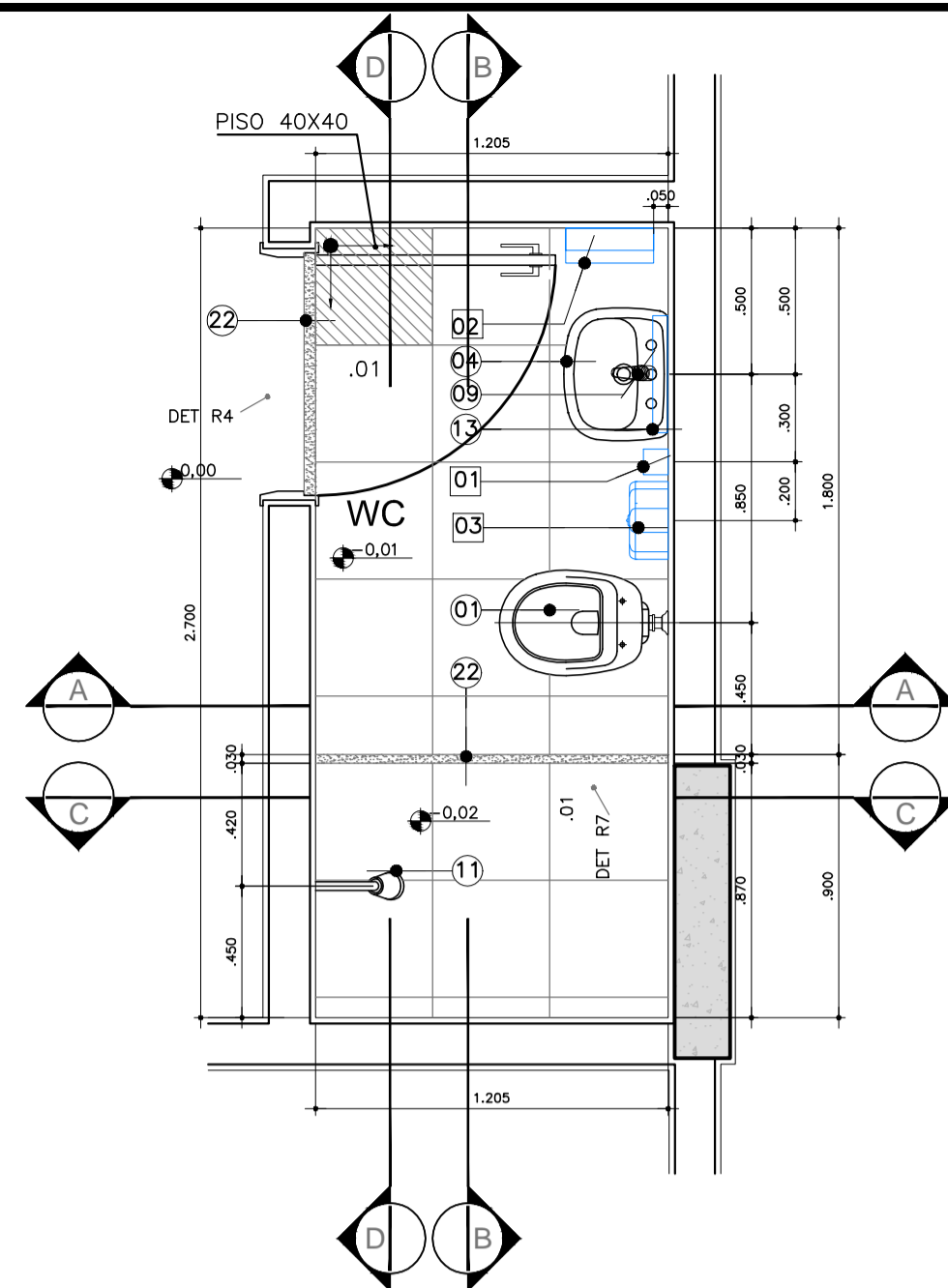
AM-01- WC PLANTÃO - TÉRREO QUANTIDADE : 1 ESC.: 1:25
