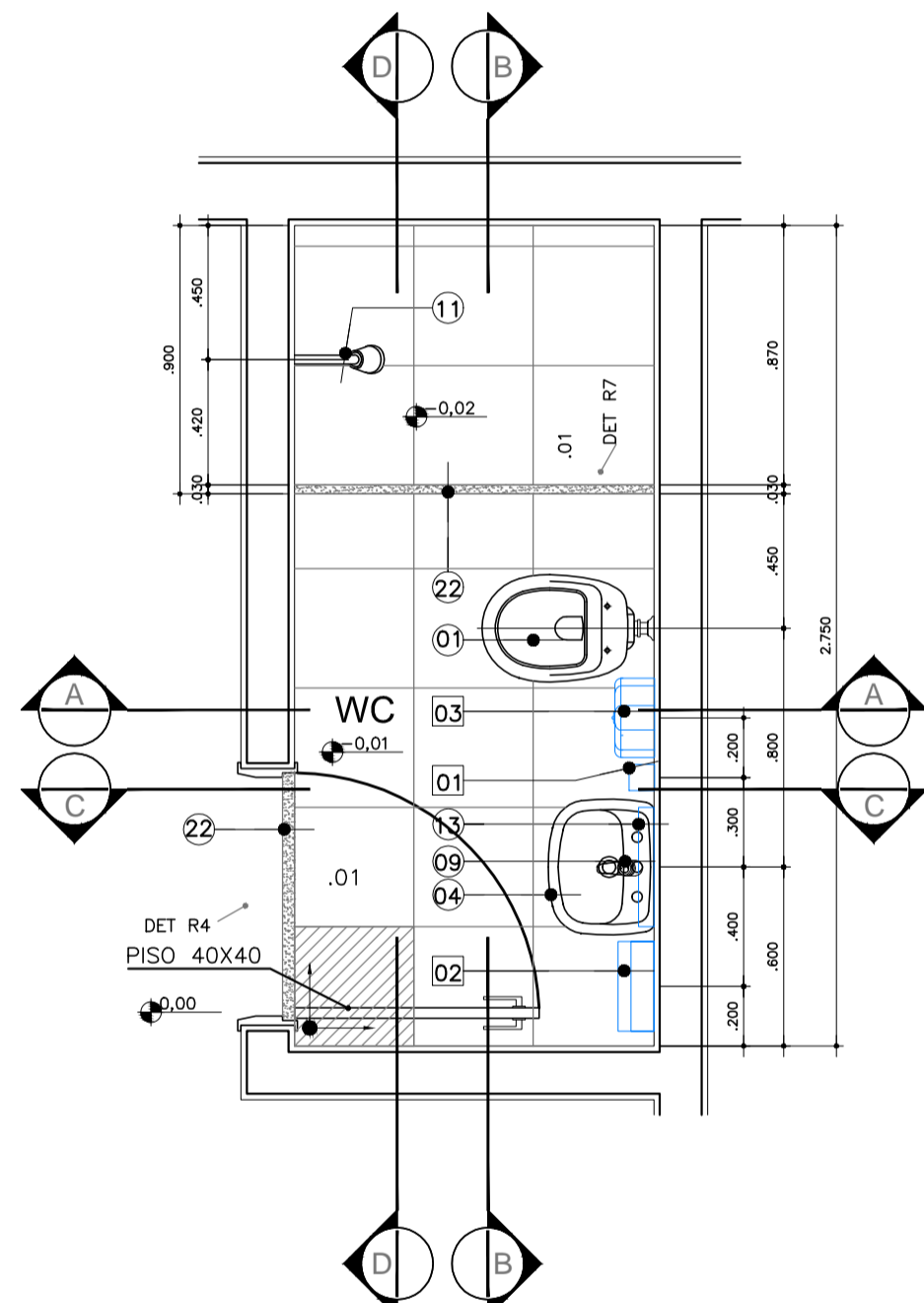
AM-02- WC PLANTÃO - TÉRREO QUANTIDADE : 1 ESC.: 1:25
