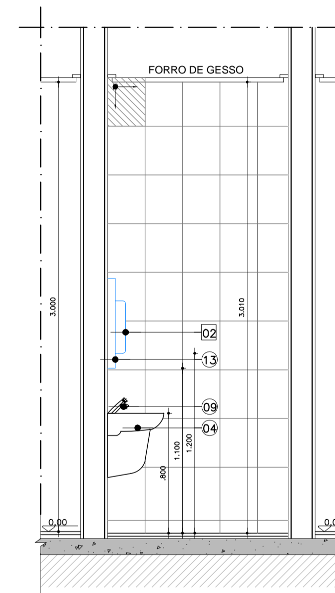
CORTE CC ESCALA 1:25 AM-01- WC PLANTÃO - TÉRREO
