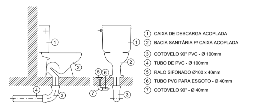
DETALHE - vaso sanitário com caixa de descarga acoplada ESC: 1/20
