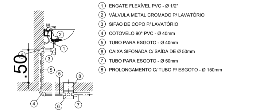
DETALHE - lavatório ESC: 1/20
