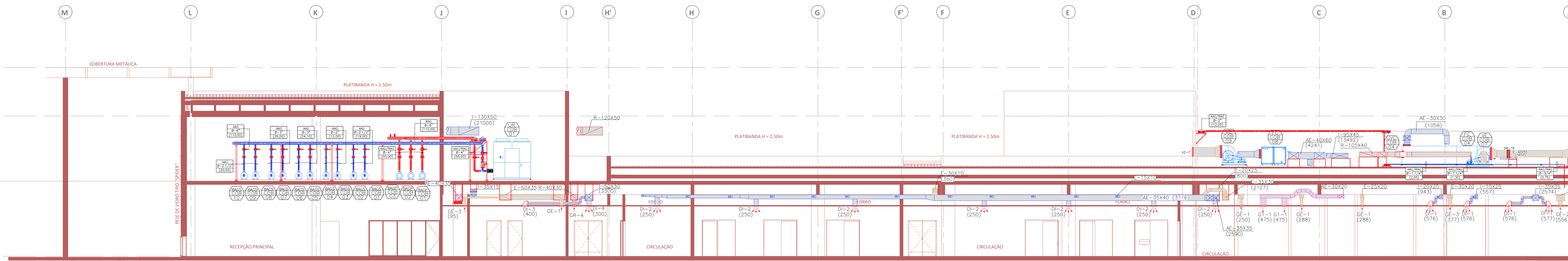
CORTE-C3 ESC: 1/100
