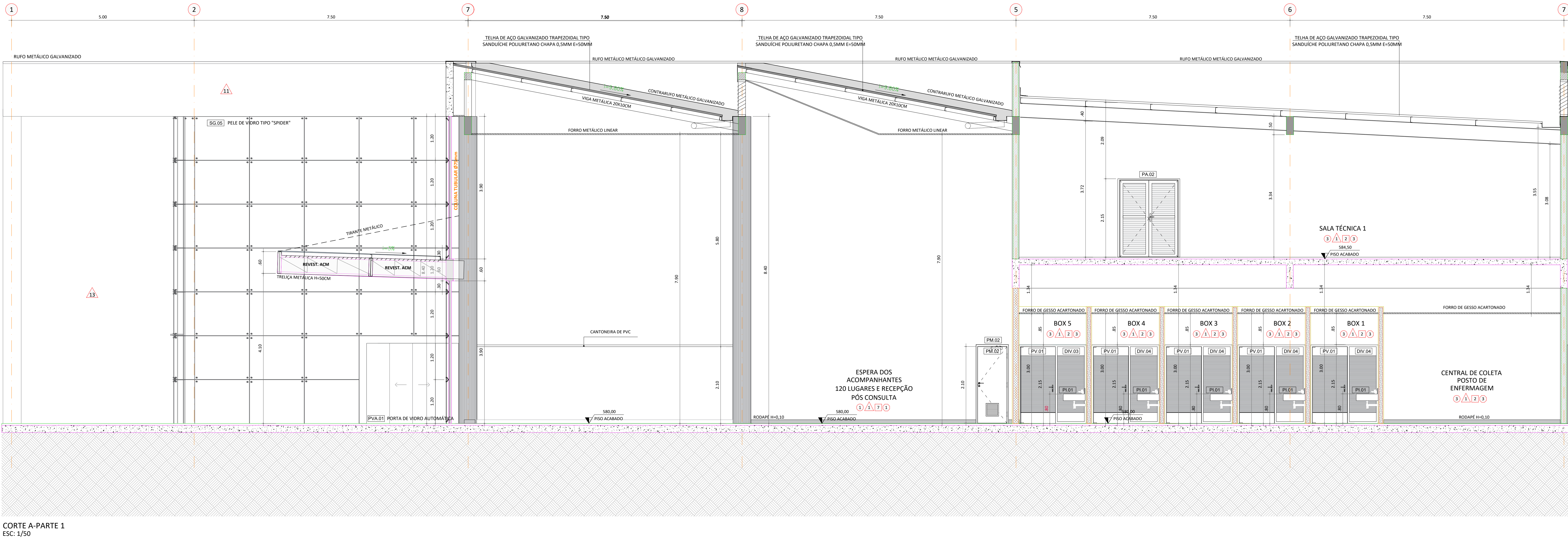
CORTE A-PARTE 1 ESC: 1/50
