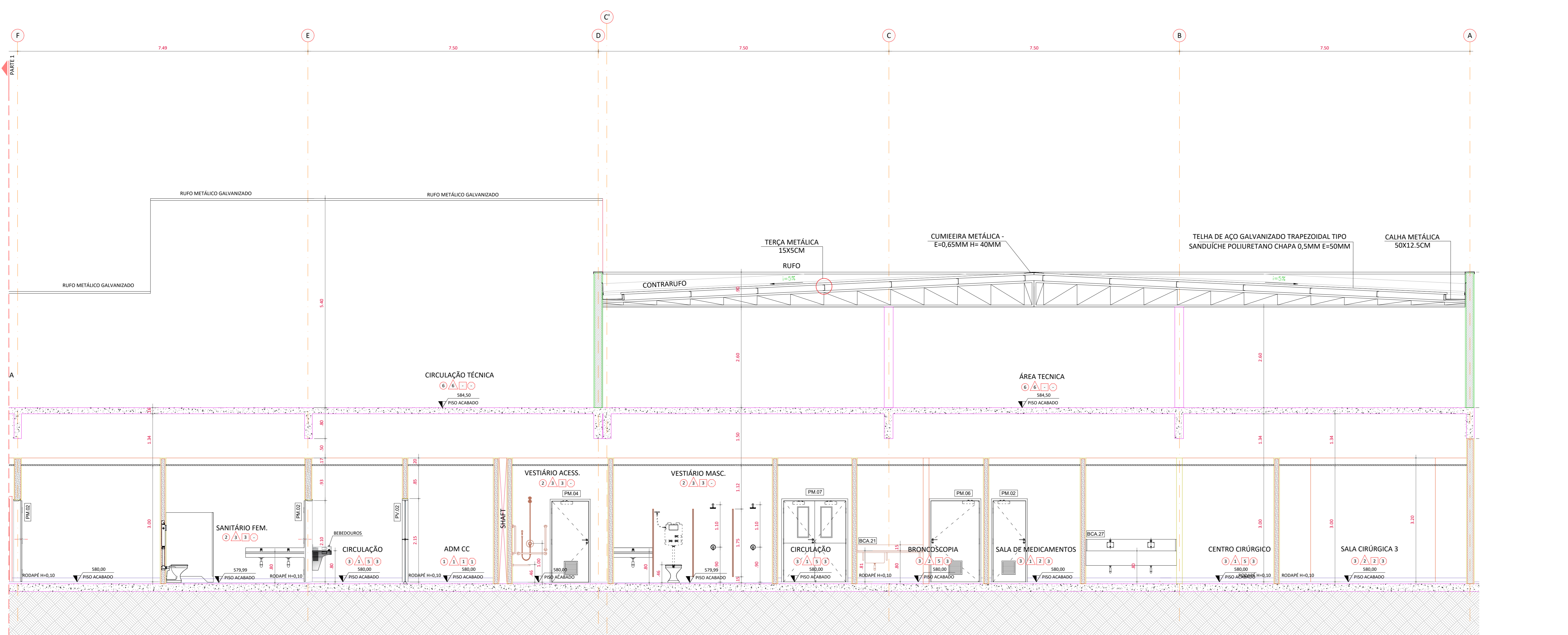
CORTE E-PARTE 2 ESC: 1/50
