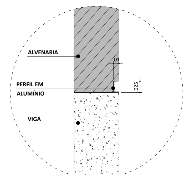
DETALHE 1 - FRISO ESC: 1/5
