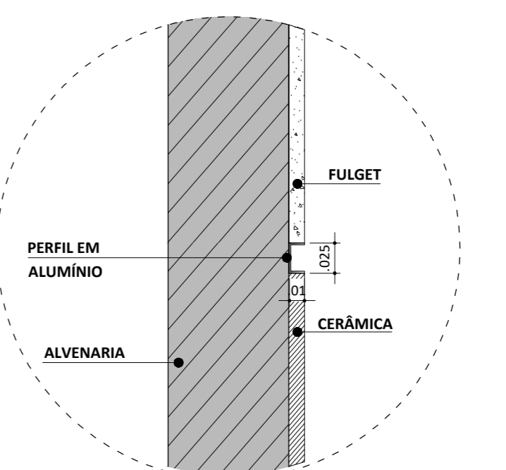
DETALHE 2 - FRISO ESC: 1/5
