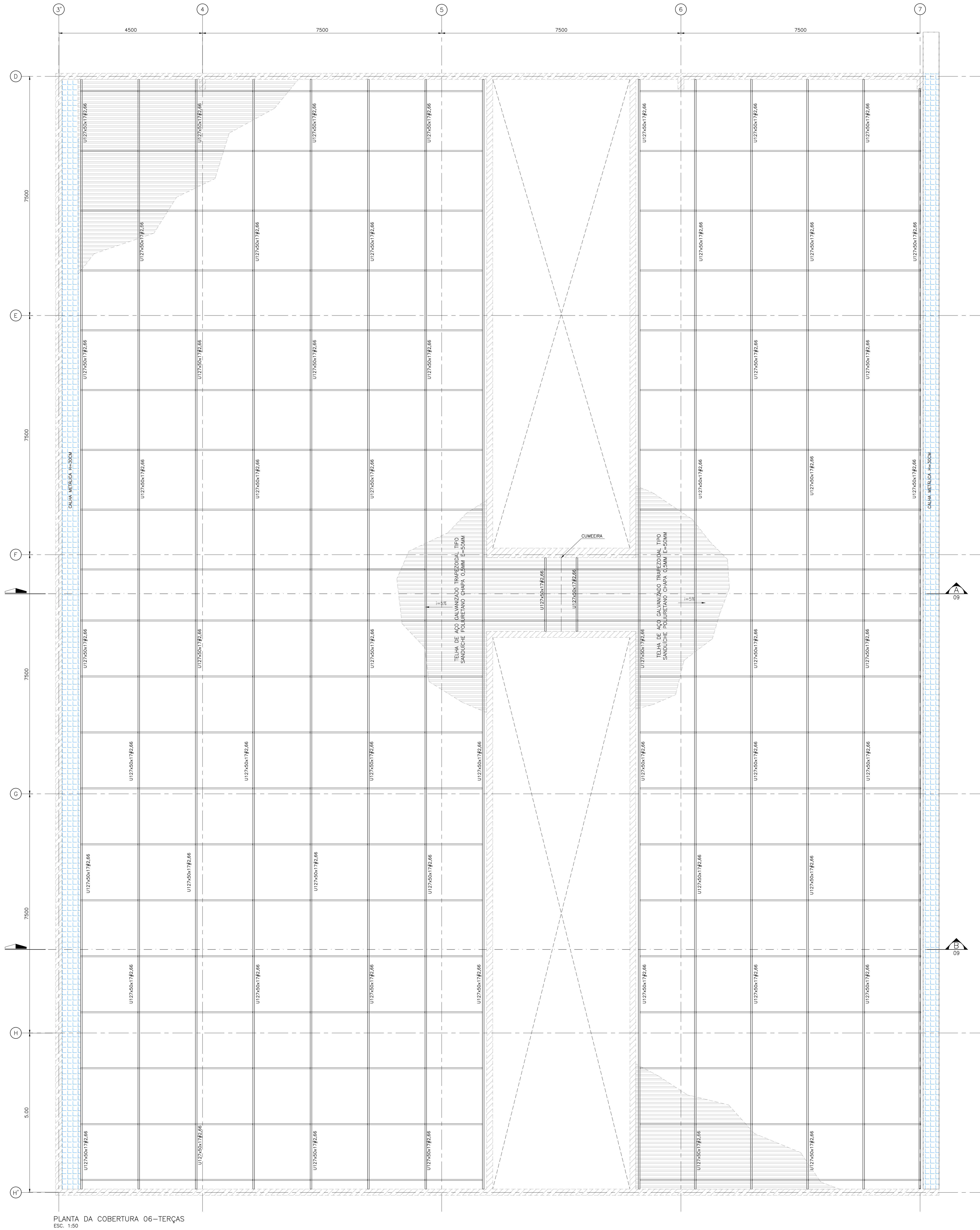
PLANTA DA COBERTURA 06-TERÇAS ESC. 1:50
