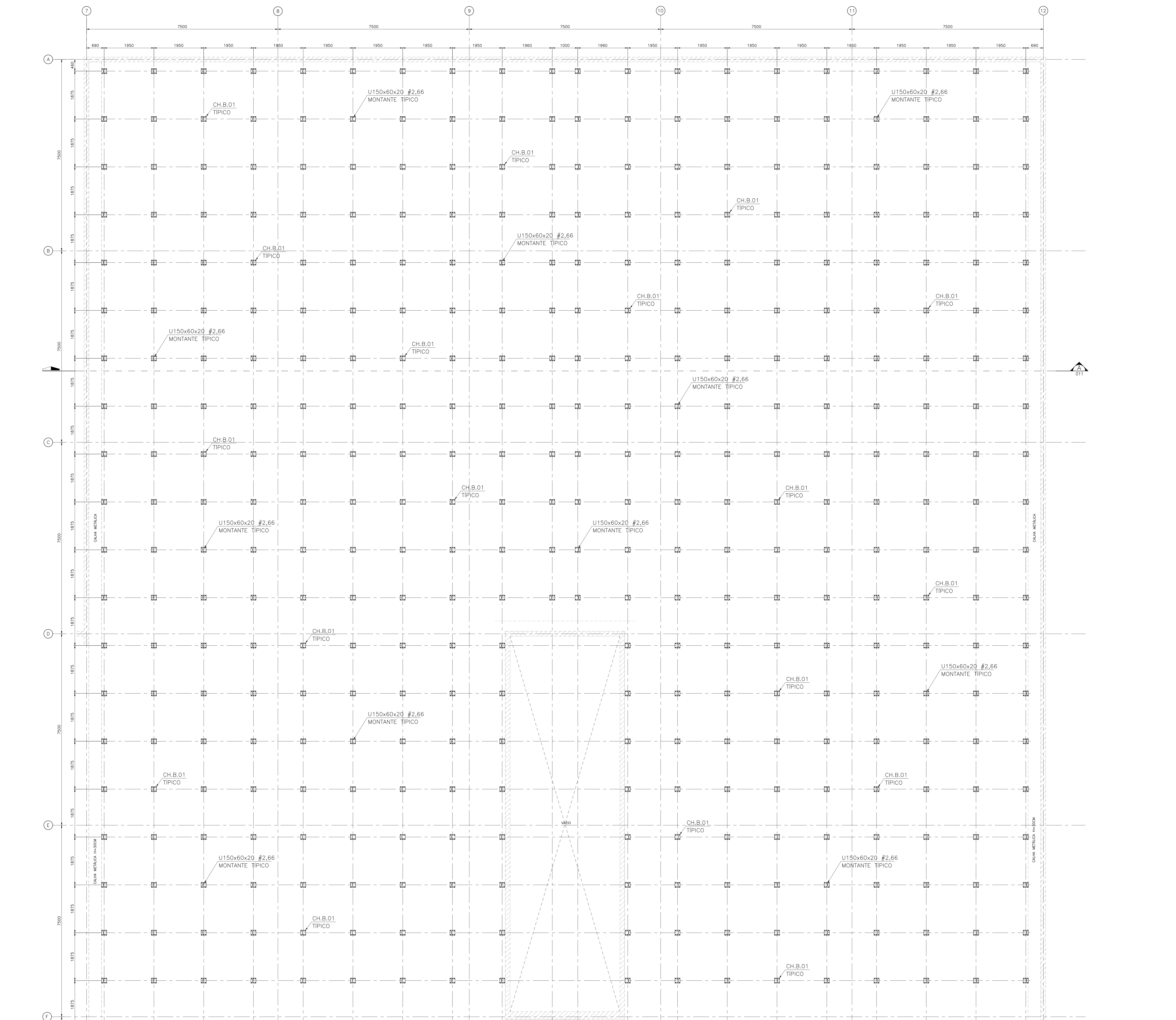
PLANTA DA COBERTURA 07 - LOCAÇÃO DAS BASES ESC: 1:50
